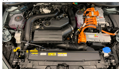
Двигателно отделение
